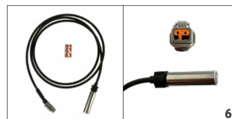
Deutsch DTM06-2S / Straight
