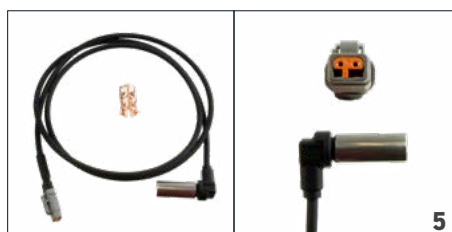
Deutsch DTM06-2S / 90 Degree
